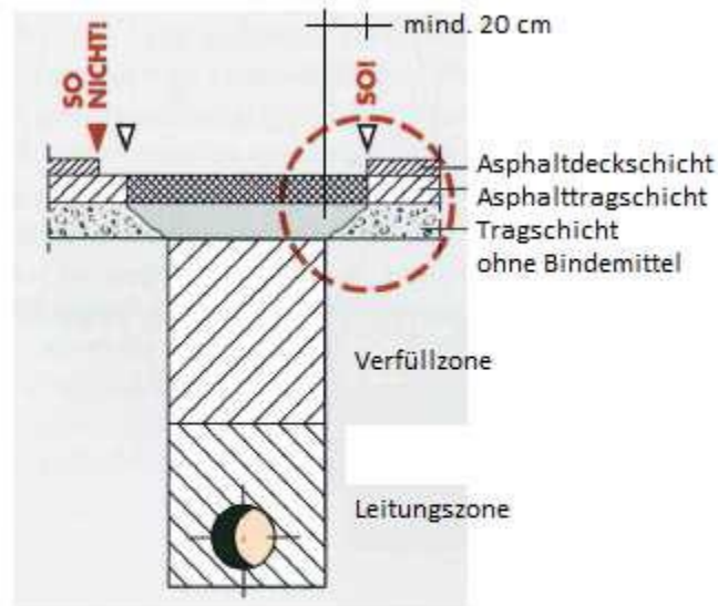
Abtreppung der Asphalttschichten (Rücknahme/Rückschnitt)
